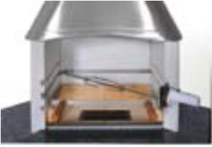
Úhlopříčný nosič grilovací jehly, grilovací jehla dl. 65 cm, motorek
